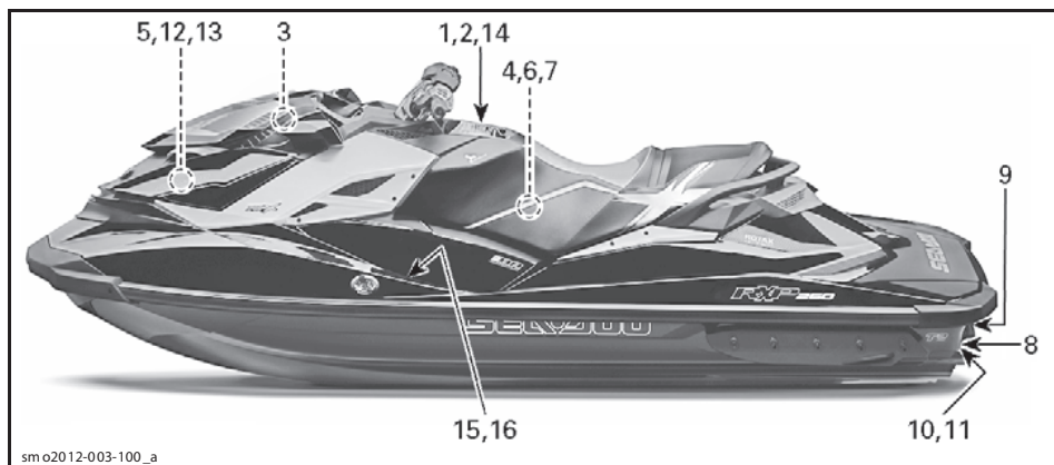
РАСПОЛОЖЕНИЕ НА ГИДРОЦИКЛЕ ПРЕДУПРЕЖДАЮЩИХ ТАБЛИЧЕК
