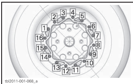
ПОСЛЕДОВАТЕЛЬНОСТЬ ФИНАЛЬНОГО ЭТАПА ЗАТЯЖКИ
