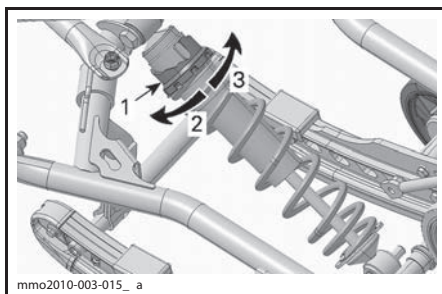
РЕГУЛЯТОР КУЛАЧКОВОГО ТИПА — АМОРТИЗАТОР HRG™
