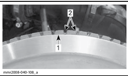
ПРЕДВАРИТЕЛЬНАЯ УСТАНОВКА 1. Кромка ведомого шкива 2. Зубцы на внешней поверхности ремня
