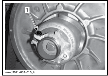
1. Фиксирующий болт
