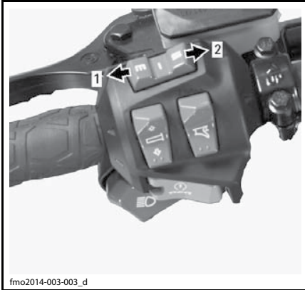
МНОГОФУНКЦИОНАЛЬНЫЙ ПЕРЕКЛЮЧАТЕЛЬ 1. Как кнопка MODE 2. Как кнопка SET
