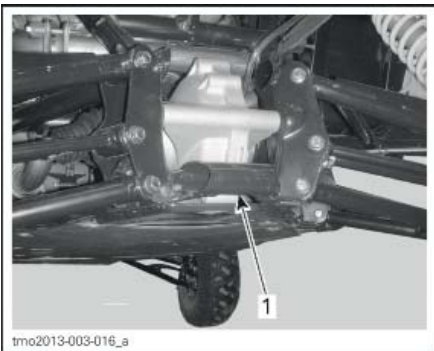
ЗАДНЯЯ ЧАСТЬ МОТОВЕЗДЕХОДА 1. Место установки гидравлического домкрата
