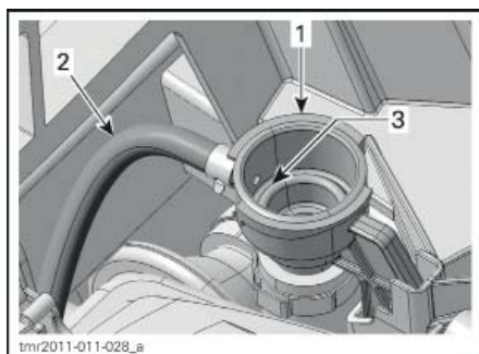
1. Горловина для заправки системы охлаждения 2. Шланг расширительного бачка 3. Уровень жидкости в системе охлаждения (посадочная поверхность крышки радиатора)
