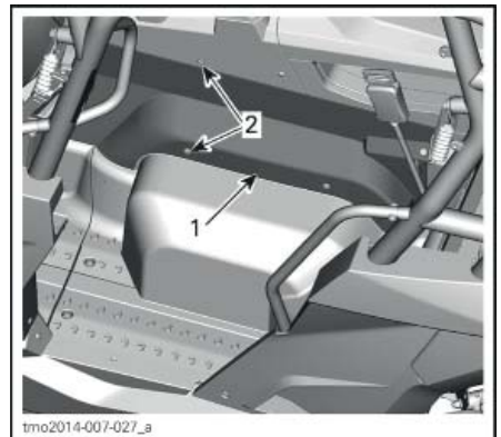
1. Задняя левая нижняя панель 2. Пластиковые фиксаторы
